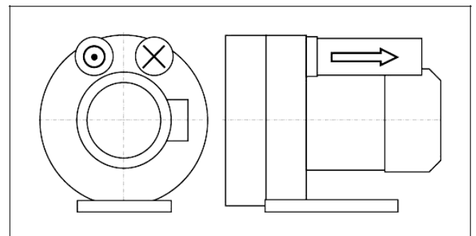
图. 4: 2RB840-7G... (双叶轮大流量规格).
