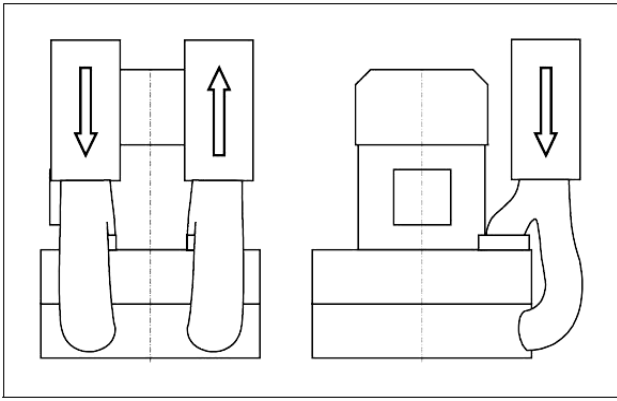
图. 7: 2RB943 (双叶轮大流量规格).
