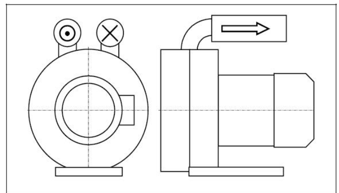
图. 5: 2RB840-7J... (双叶轮大流量规格).
