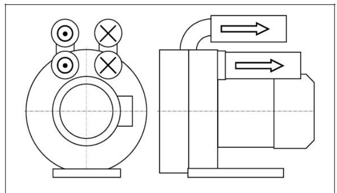
图. 6: 2RB840-7L... (双叶轮大流量规格).
