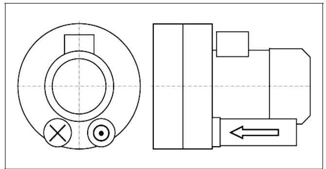
图. 3: 2RB740 (双叶轮规格)
